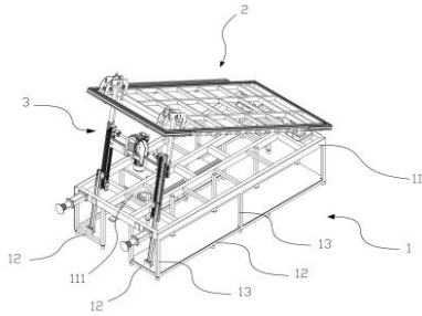
<모노레일용 수평조절장치(제 1 형태)>
