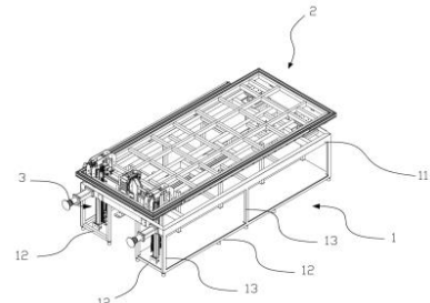
<모노레일용 수평조절장치(제 2 형태)>
